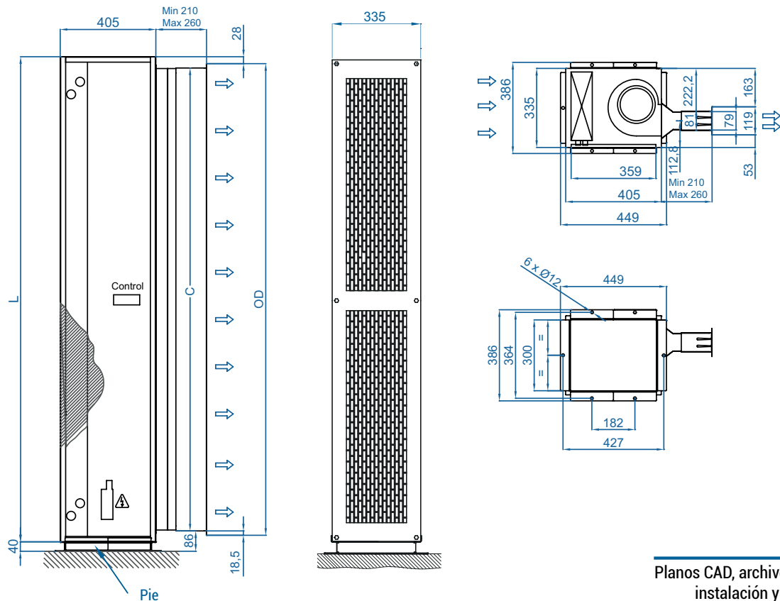
Instalación vertical
