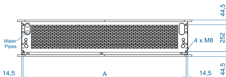
Instalación vertical
