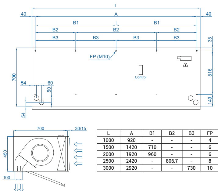
Instalación horizontal
