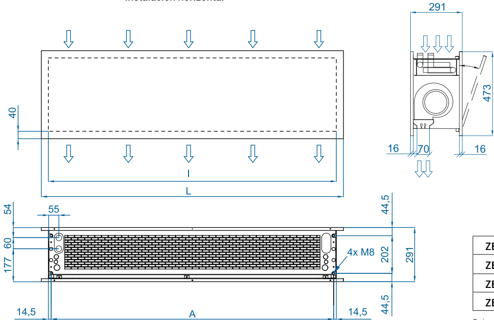
Instalación horizontal
