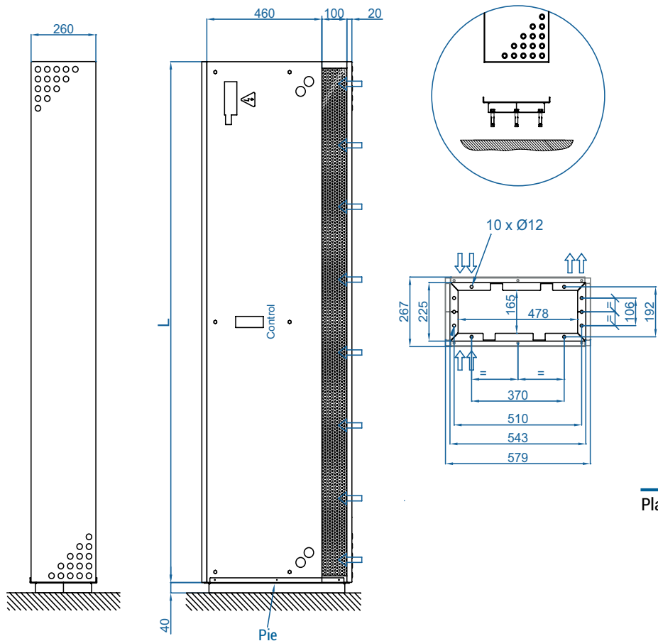
Instalación vertical
