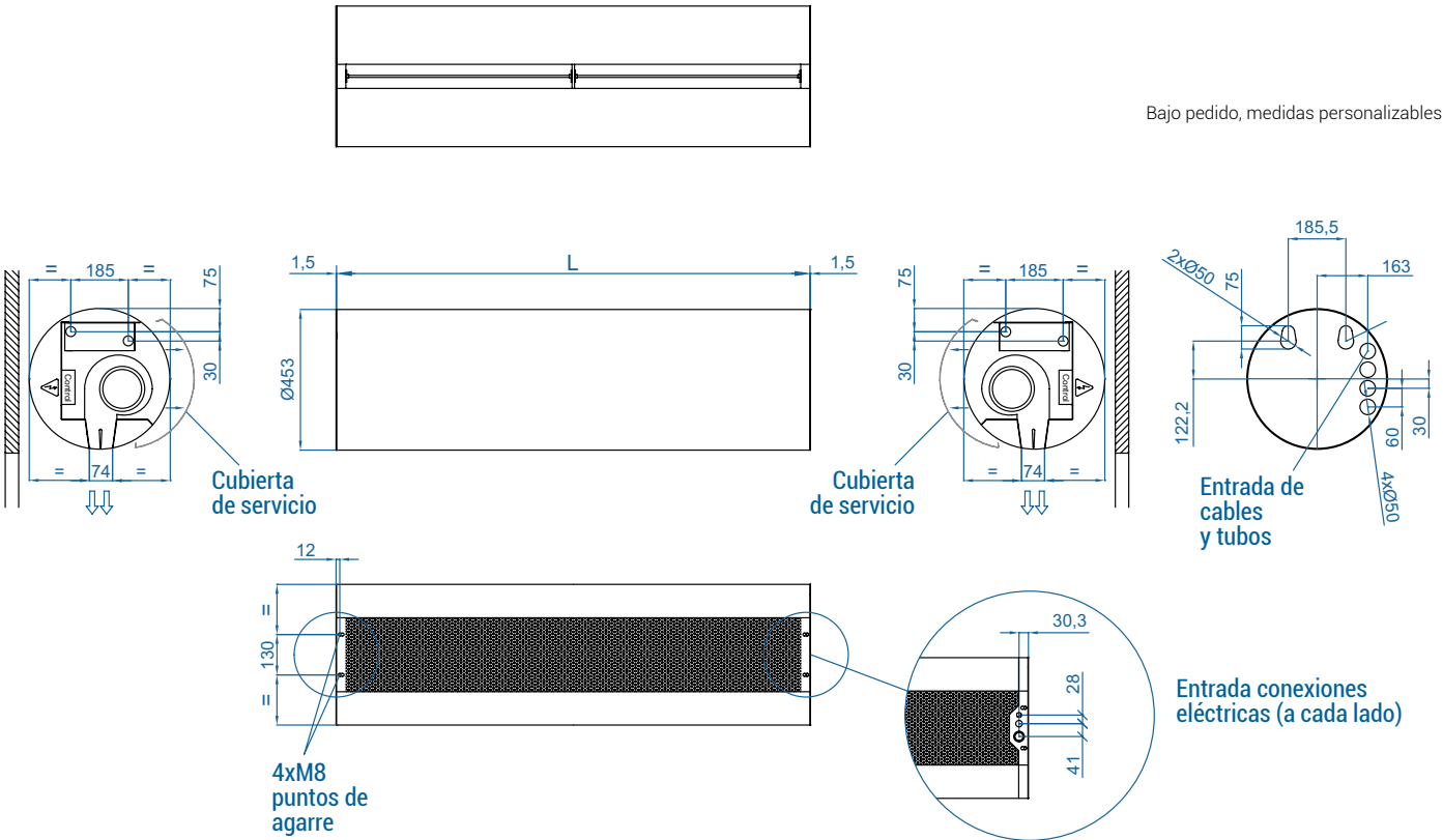
Instalación vertical
