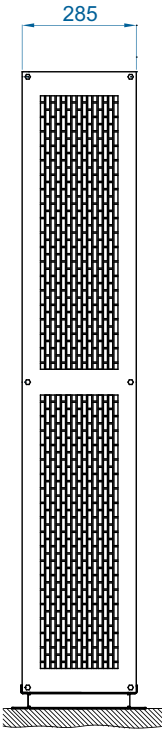
Instalación vertical
