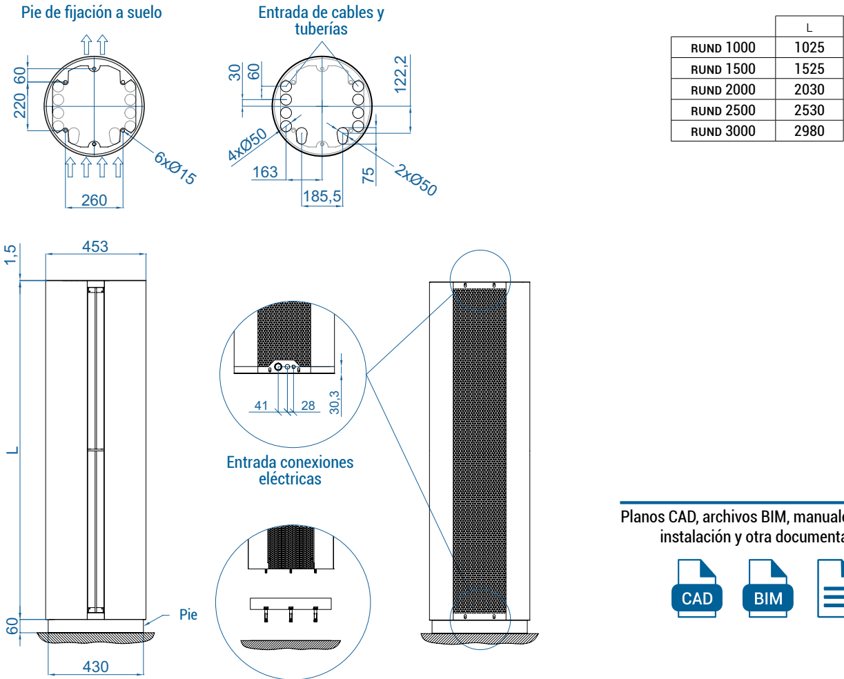
Instalación vertical
