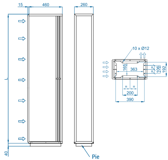
Instalación vertical
