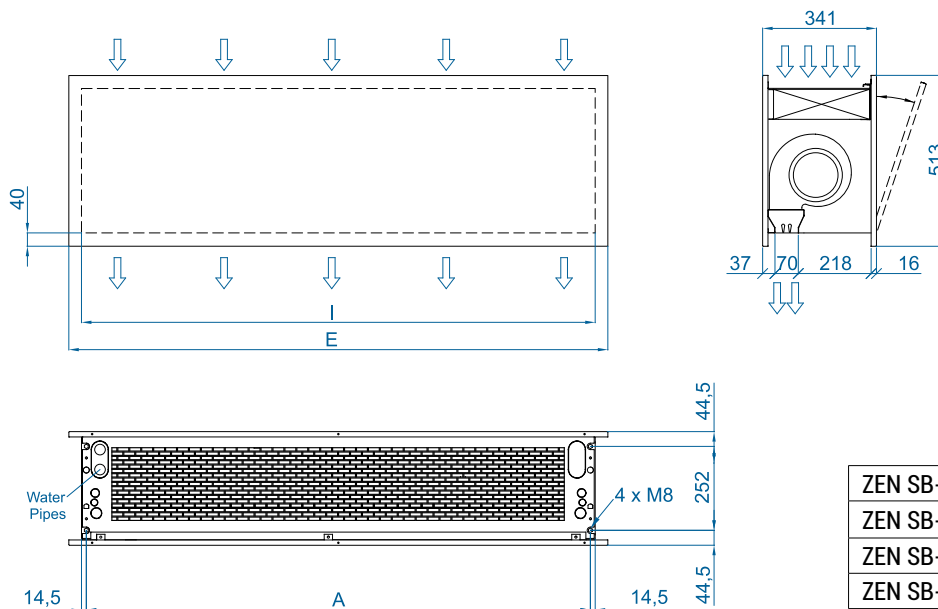
Instalación horizontal
