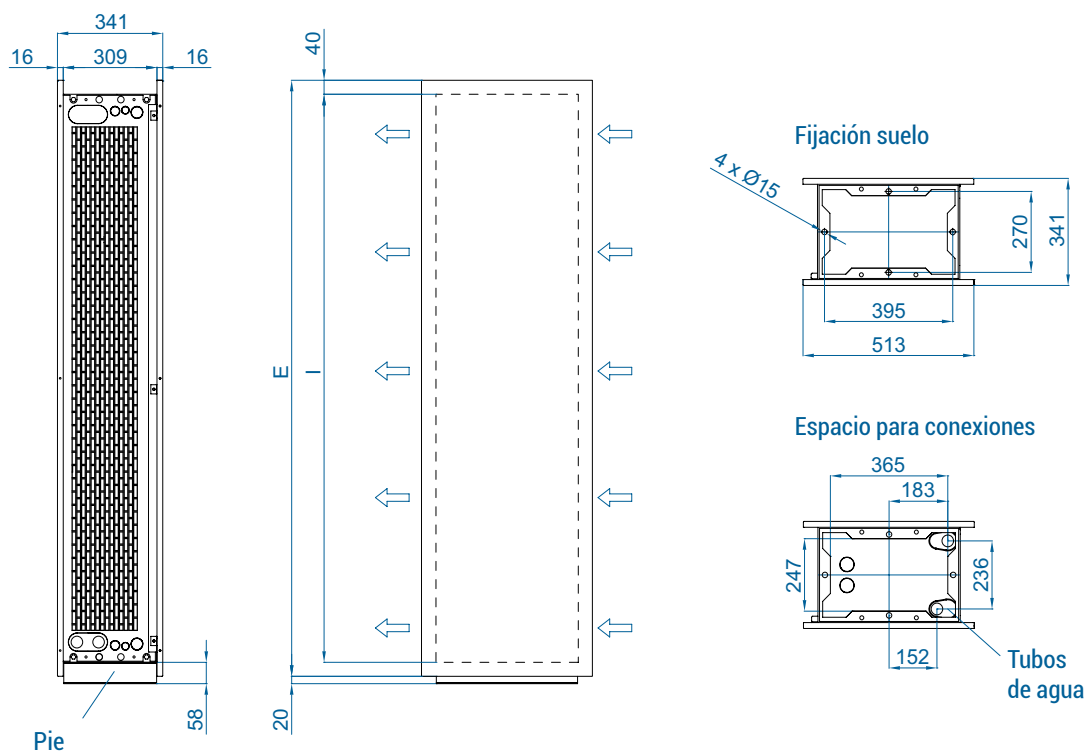
Instalación vertical
