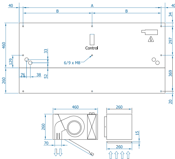
Instalación vista en falso techo
