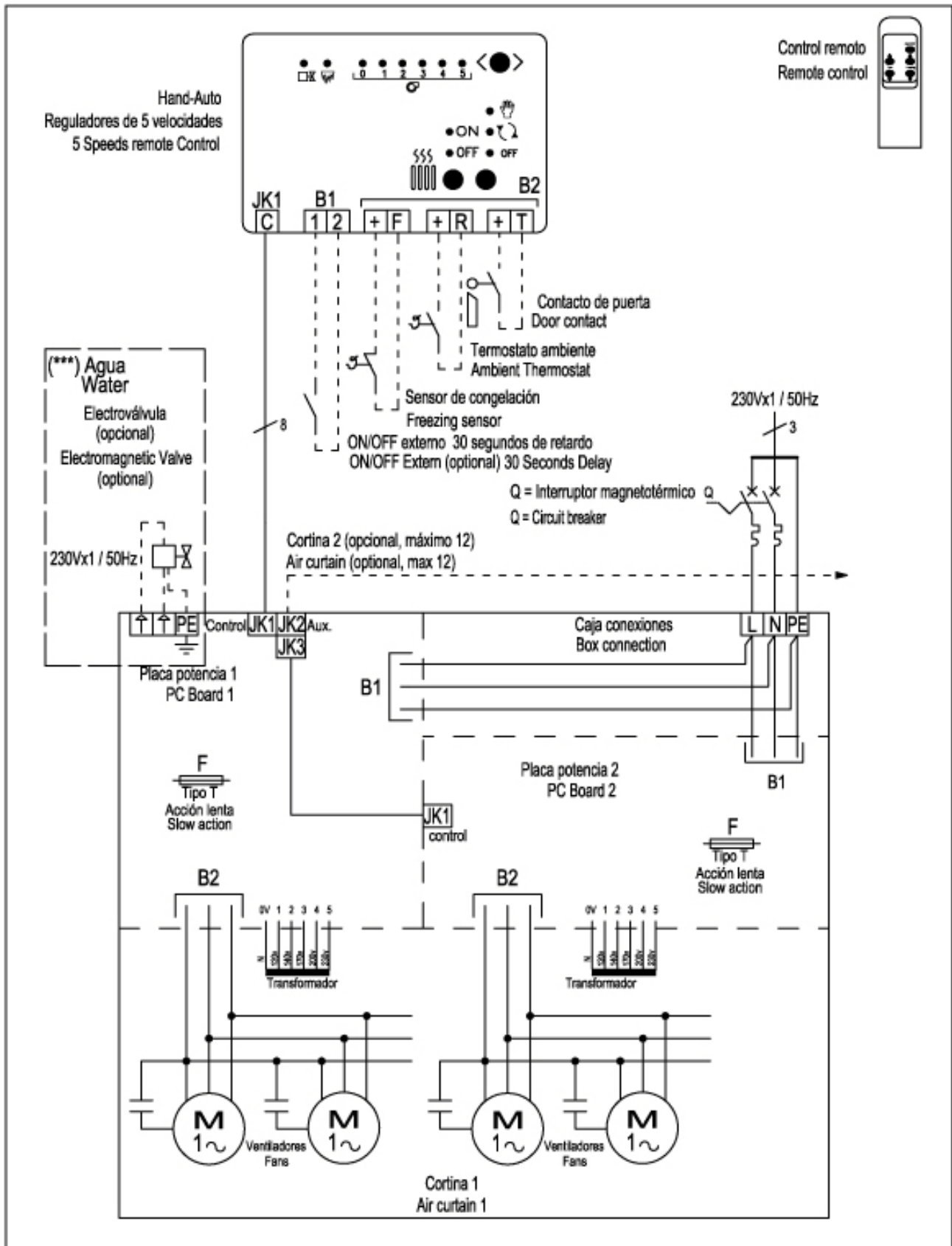
ESQUEMAS ELÉCTRICOS CORTINA DE AIRE WIRING DIAGRAMS OF AIR CURTAIN CONTROLADOR 5 VELOCIDADES Hand-Auto AGUA O AIRE L 2000-2500-3000, XL 1500-2000 WATER AND ONLY AIR, Hand-Auto CONTROLLER 5 SPEEDS. L 2000-2500-3000, XL 1500-2000 Pág./Page 1 de/of 1 Doc. AIRDOE09867 R12 - 17/02/16
