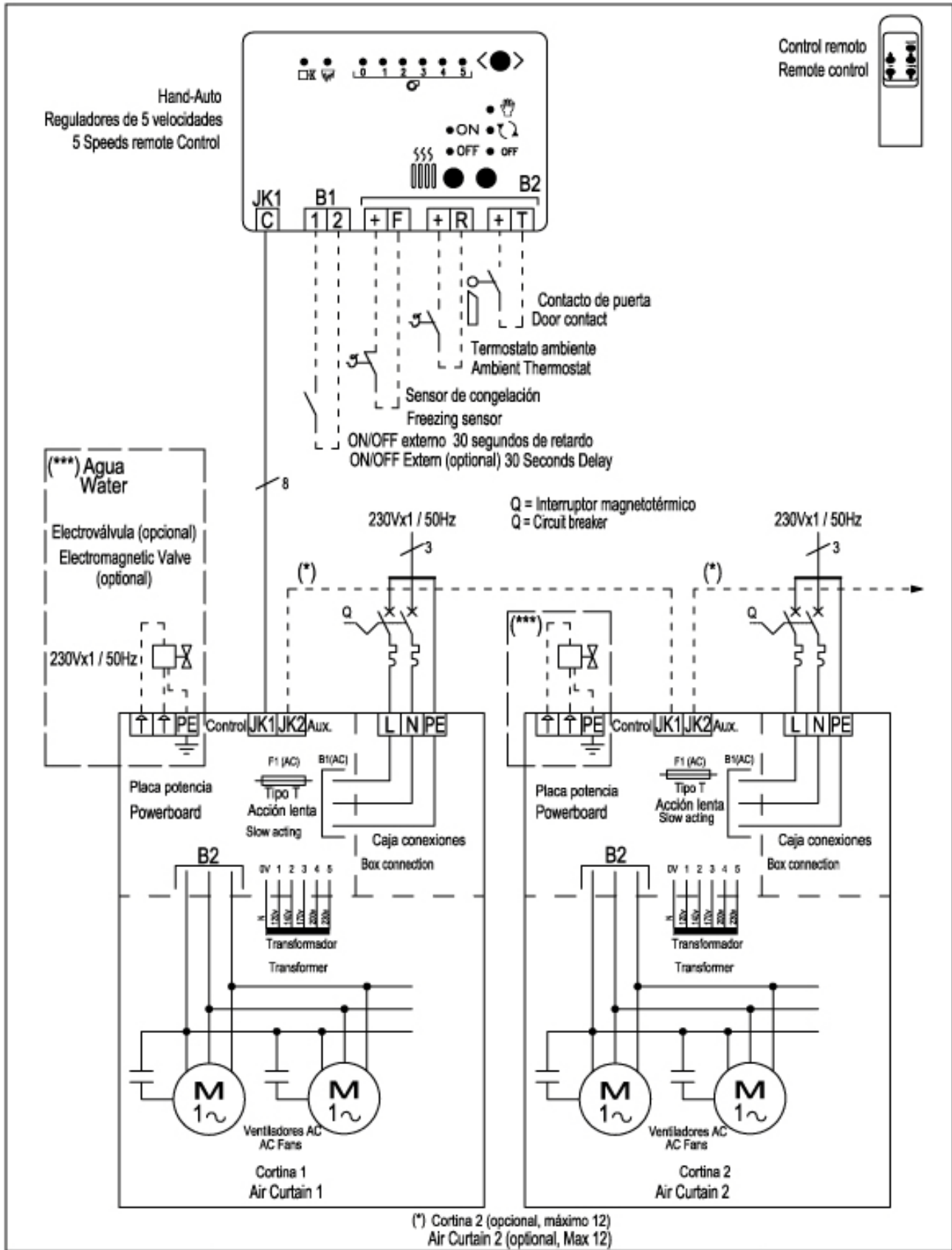
ESQUEMAS ELÉCTRICOS CORTINA DE AIRE VENTILADORES AC/EC WIRING DIAGRAMS OF AIR CURTAIN AC/EC FANS CONTROLADOR Hand-Auto AGUA O AIRE L 1000-1500, XL 1000 WATER AND ONLY AIR, CONTROLLER 5 SPEEDS. L 1000-1500, XL 1000
