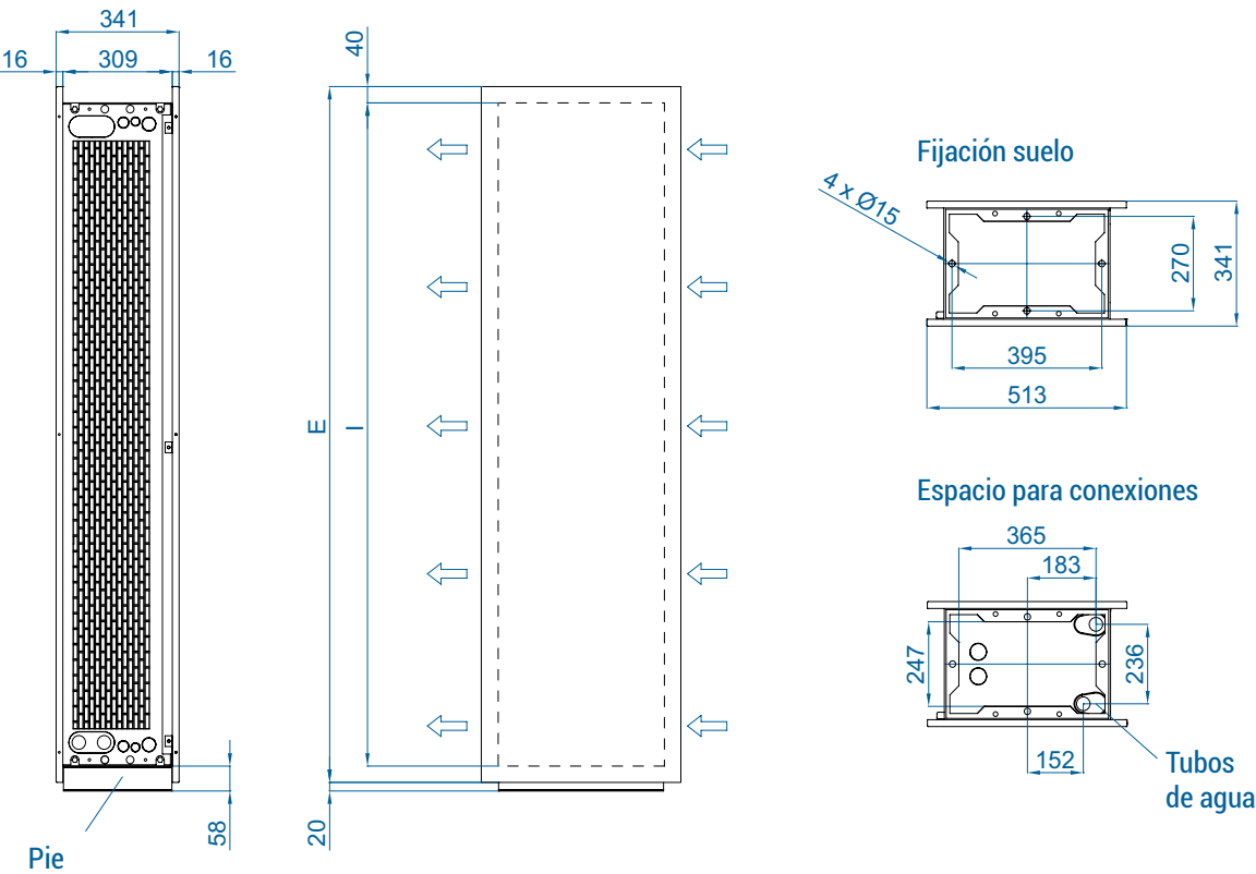
Instalación vertical
